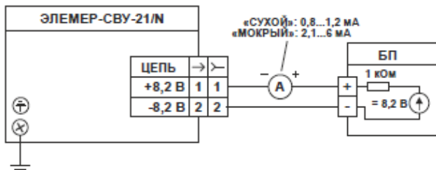
Рисунок В.4 - Схема электрическая подключения сигнализаторов ЭЛЕМЕР-СВУ-21 и ЭЛЕМЕР-СВУ-21А с кодом при заказе N (с выходным сигналом NAMUR)
